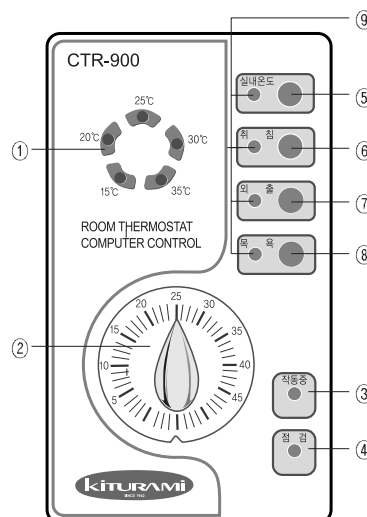
Регулятор температуры в помещении (CTR-900)
